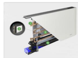
SLR Smart model: 1) elektrotermički osigurač; 2) spiralni radijatorski grijač; 3) izmjenjivač; 4) visoko učinkoviti tangencijalni ventilator
